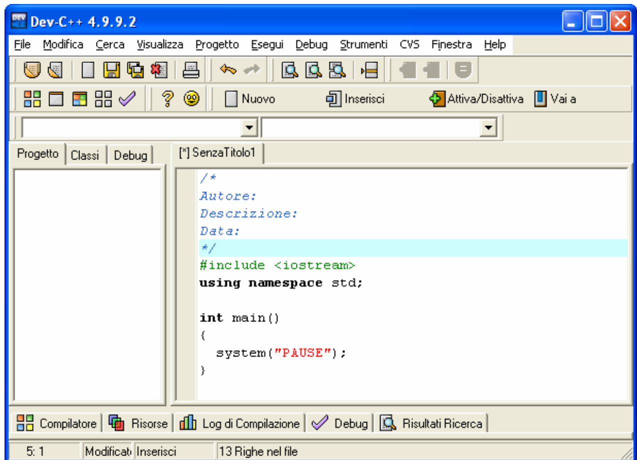
Fig. 1.2: L'IDE DevC++ 4.9.9.2
