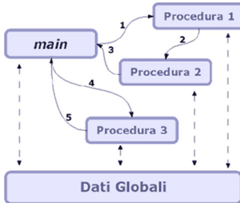
Figura 2. Flusso di un programma con programmazione procedurale
