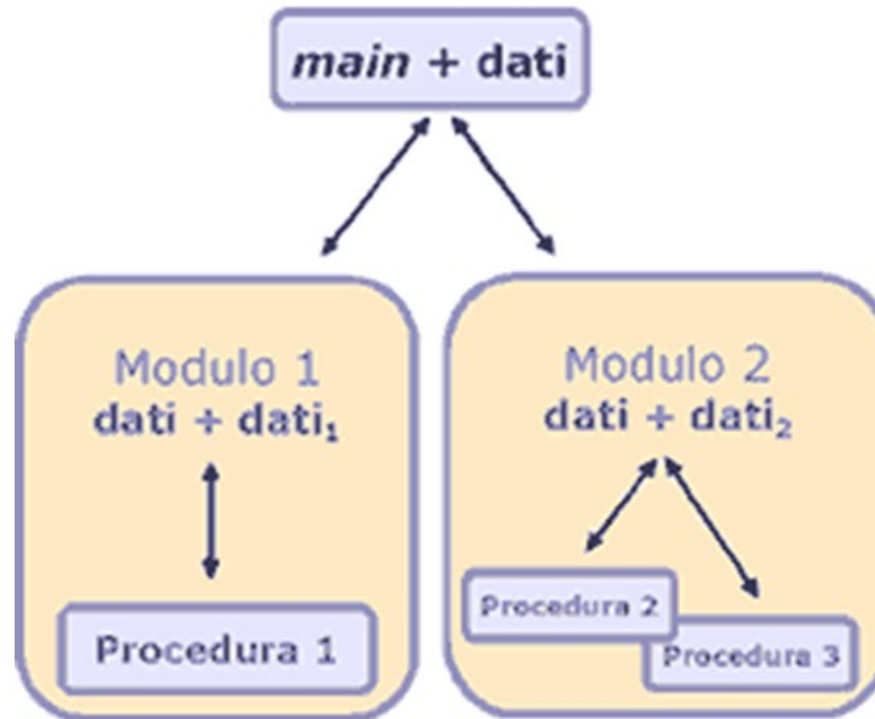
Figura 3. Struttura di un programma «modulare»
